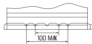
Bodenleiste B13
